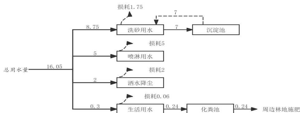
图 2-2 2#砂石加工场水平平衡图 (m³/d)
