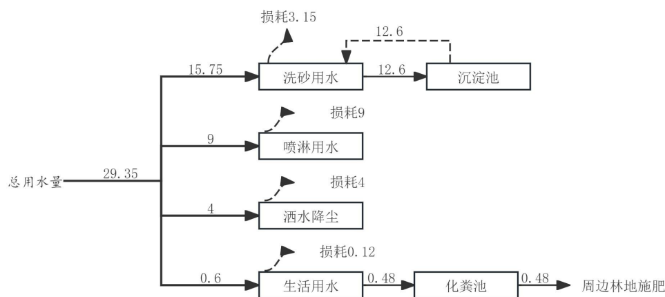
图 2-3 项目总水平平衡图 (m³/d)
