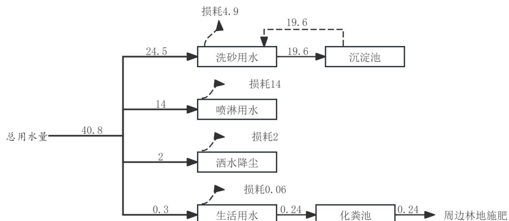
图 2-2 德兰村至那连村可采区（3/4）砂石加工场水平衡图 (m³/d)
