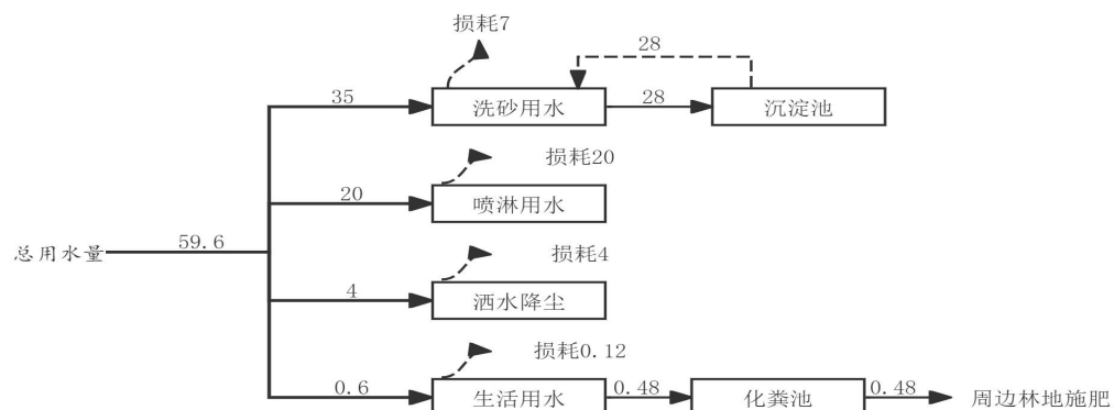
图 2-3 项目总水平衡图 (m³/d)
