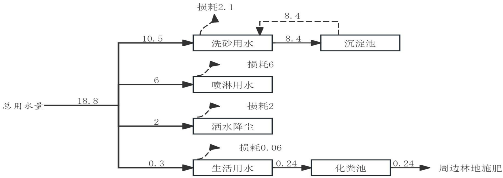
图 2-1 德兰村至那连村可采区（1/4）砂石加工场水平衡图 (m³/d)
