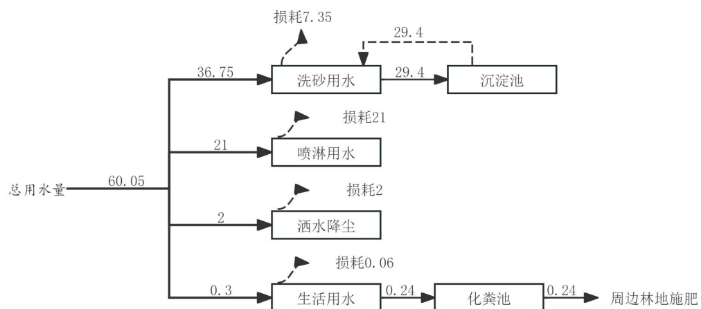
图 2-1 冲吉组可采区砂石加工场水平衡图 (m³/d)
