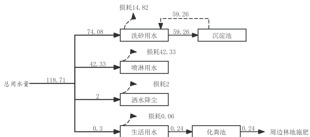
图 2-2 下坝组可采区砂石加工场水平衡图 (m³/d)
