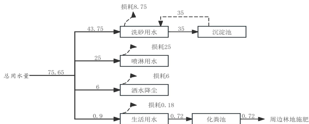
图 2-4 项目总水平衡图 (m³/d)
