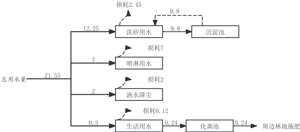
图 2-1 平木村可采区砂石加工场水平衡图 (m 3 /d)
