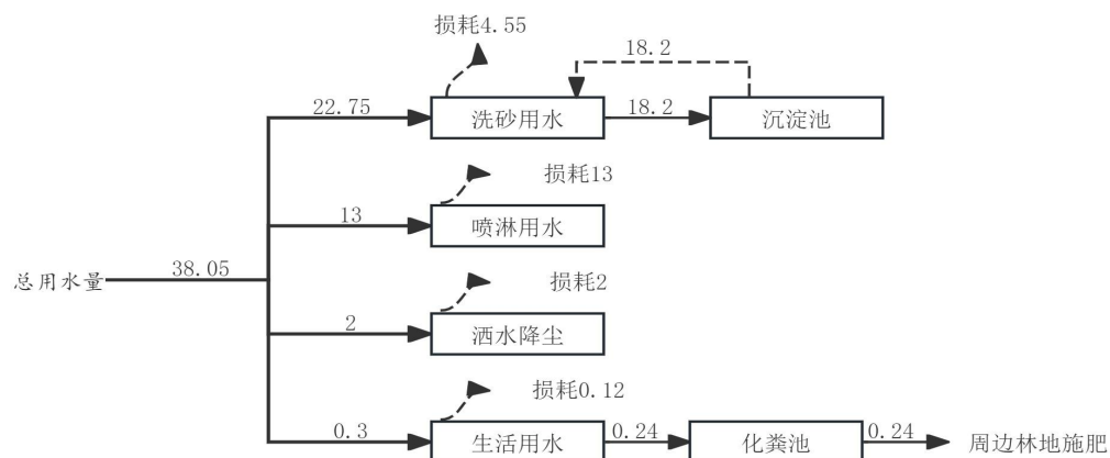
图 2-2 炮台村可采区 1#砂石加工场水平衡图 (m³/d)
