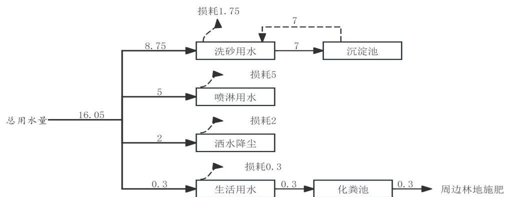
图 2-3 炮台村可采区 2#砂石加工场总水平衡图 (m³/d)
